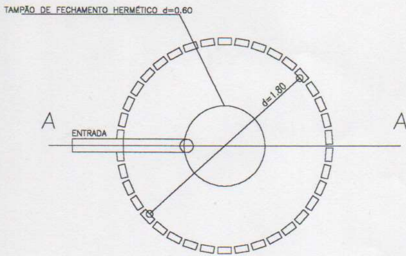
PLANTA
