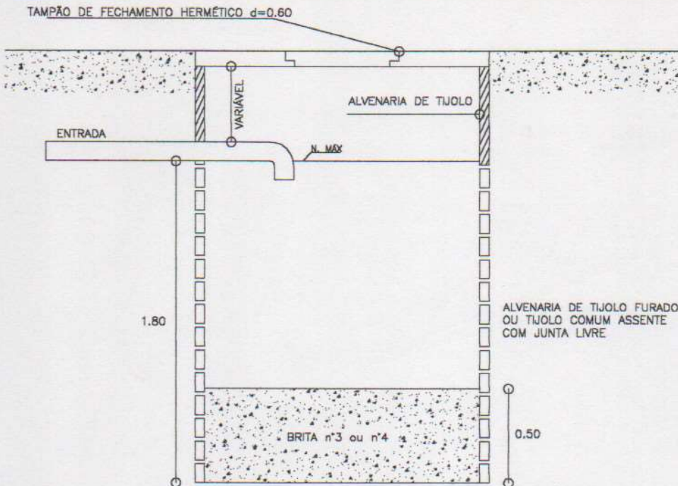
CORTE AA
