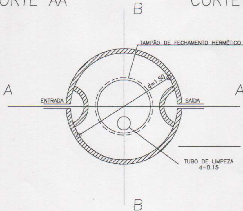
CORTE AA
